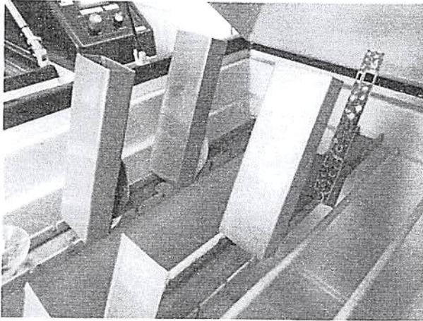
Disposição da amostra na câmara de névoa salina.
