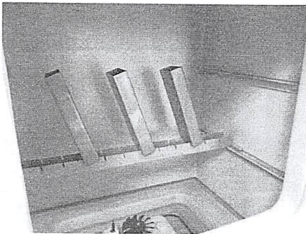
Disposição da amostra na câmara de Umidade saturada.
