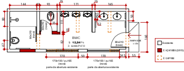
PLANTA BAIXA - Bwc Masculino ESCALA: 1/50
