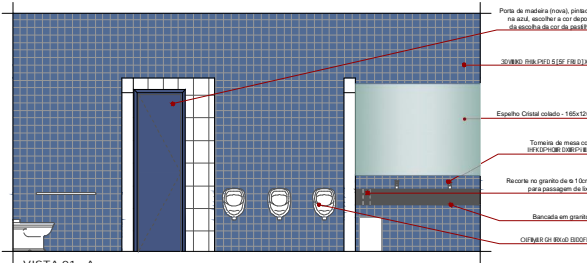
VISTA 01 - A ESCALA: 1/25
