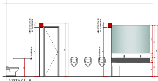
VISTA 01 - B ESCALA: 1/25
