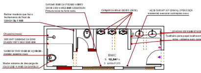
PLANTA BAIXA - Bwc Masculino ESCALA: 1/50
