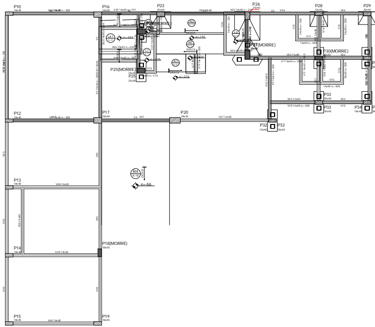
Forma do pavimento térreo escala 1:50
