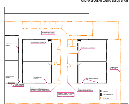
PLANTA BAIXA - Demolir ESCALA: 1/100
