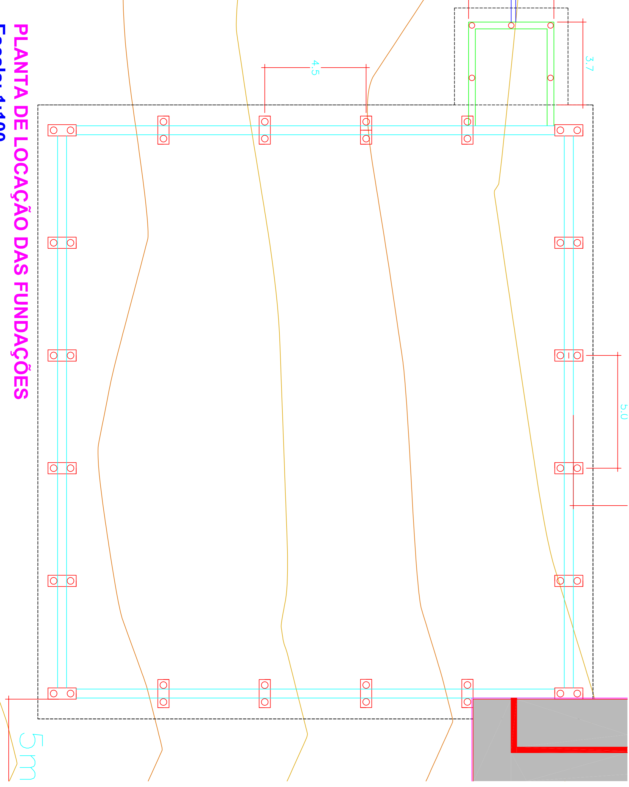
PLANTA Escala: 1:100
