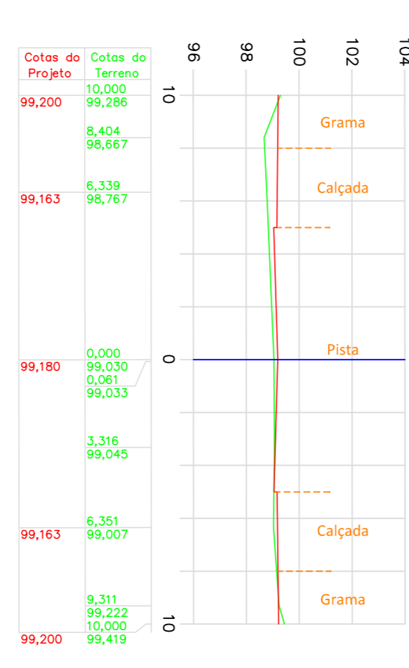
Estaca 3 Cota do terreno: 99,030 Cota do projeto: 99,180
