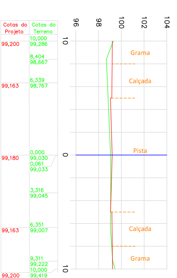
Estaca 3 Cota do terreno: 99,030 Cota do projeto: 99,180
