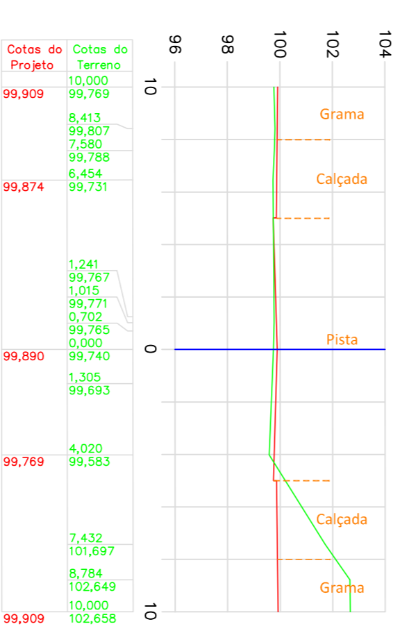
Estaca 0 Cota do terreno: 99,740 Cota do projeto: 99,890
