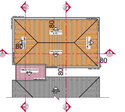
3.0 PLANTA DE COBERTURA ESCALA 1:100
