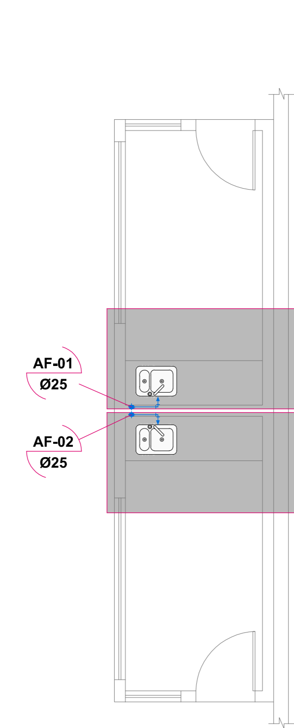
1.0 PLANTA BAIXA - Hidro ESCALA 1:50
