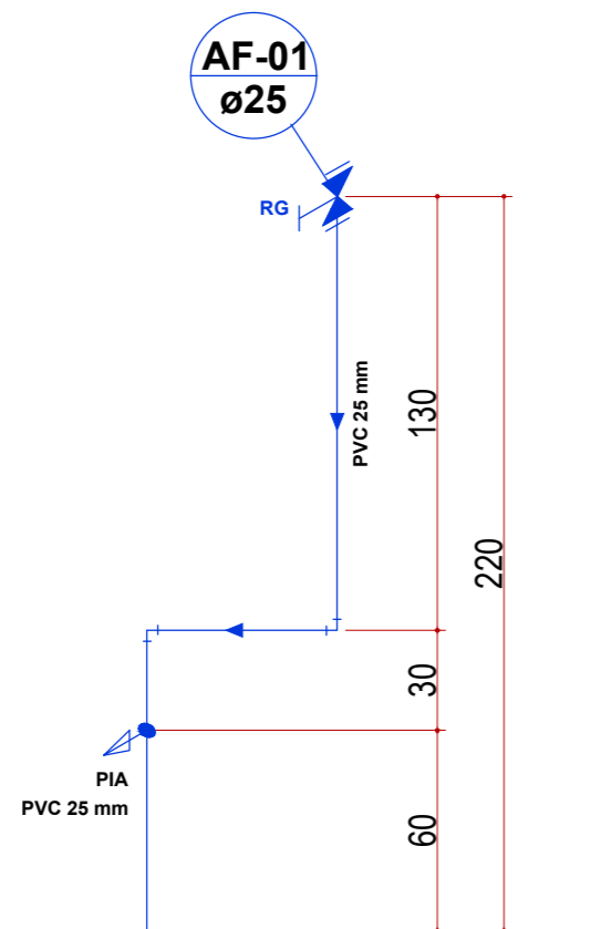
2.1 Esquema Água Fria H01 ESCALA 1:25
