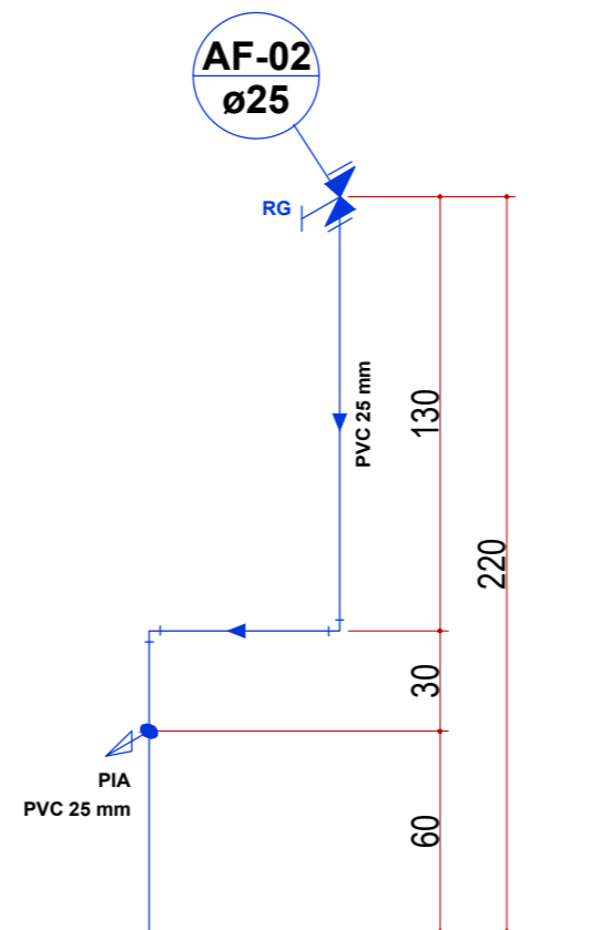
2.1 Esquema Água Fria H02 ESCALA 1:25
