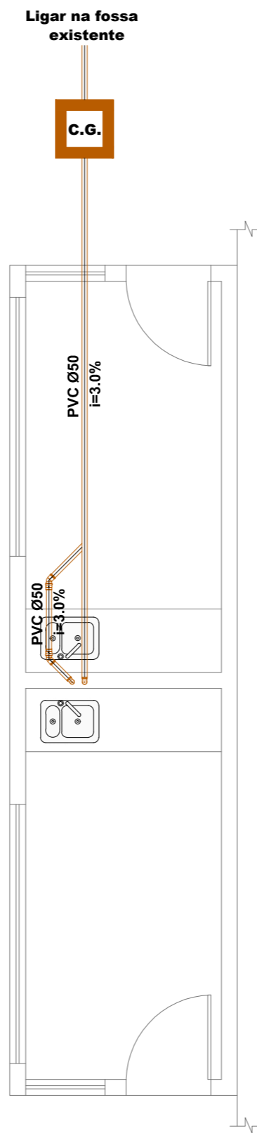
1.1 PLANTA BAIXA - Sanitário ESCALA 1:50
