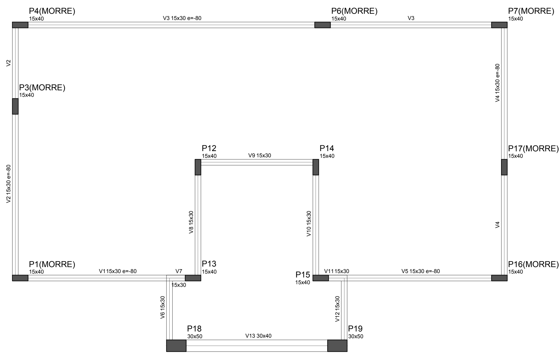
Forma do pavimento platibanda escala 1:50
