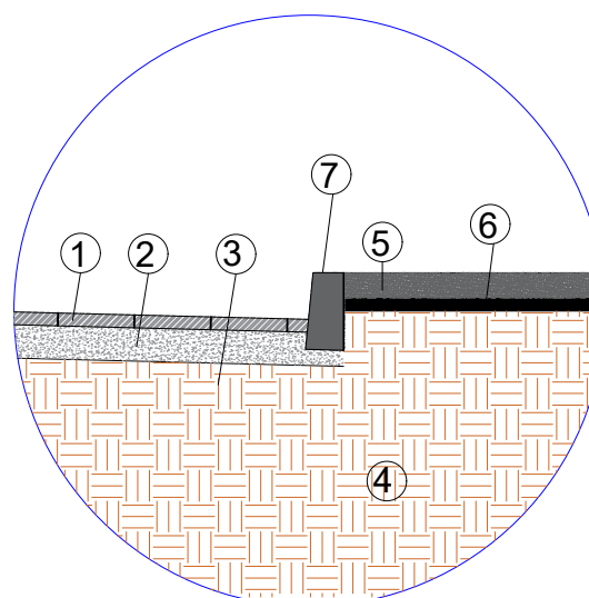
DETALHE 1
