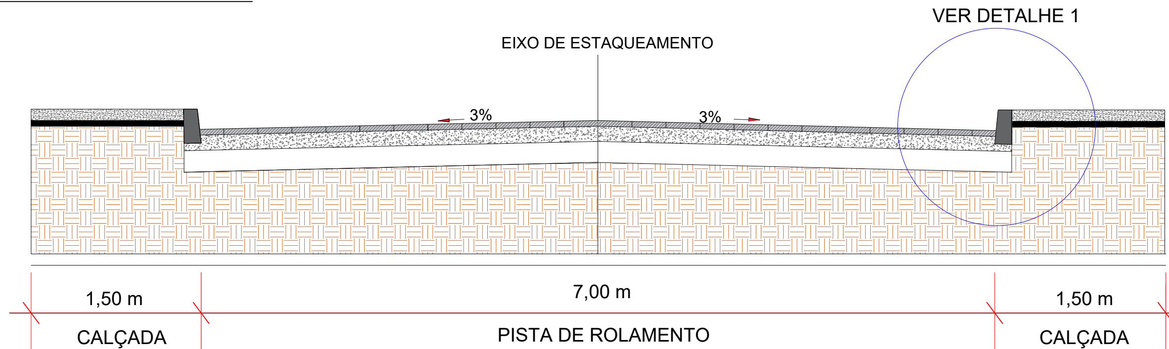
SEÇÃO TIPO SEM ESCALA
