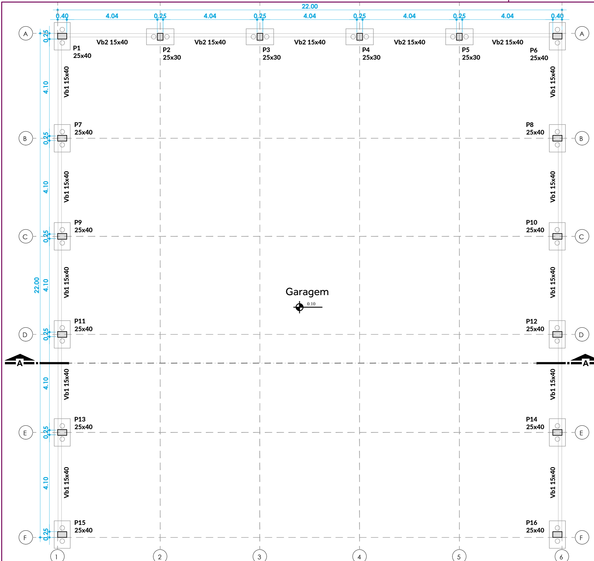
Planta de forma fundação | Esc: 1:75
