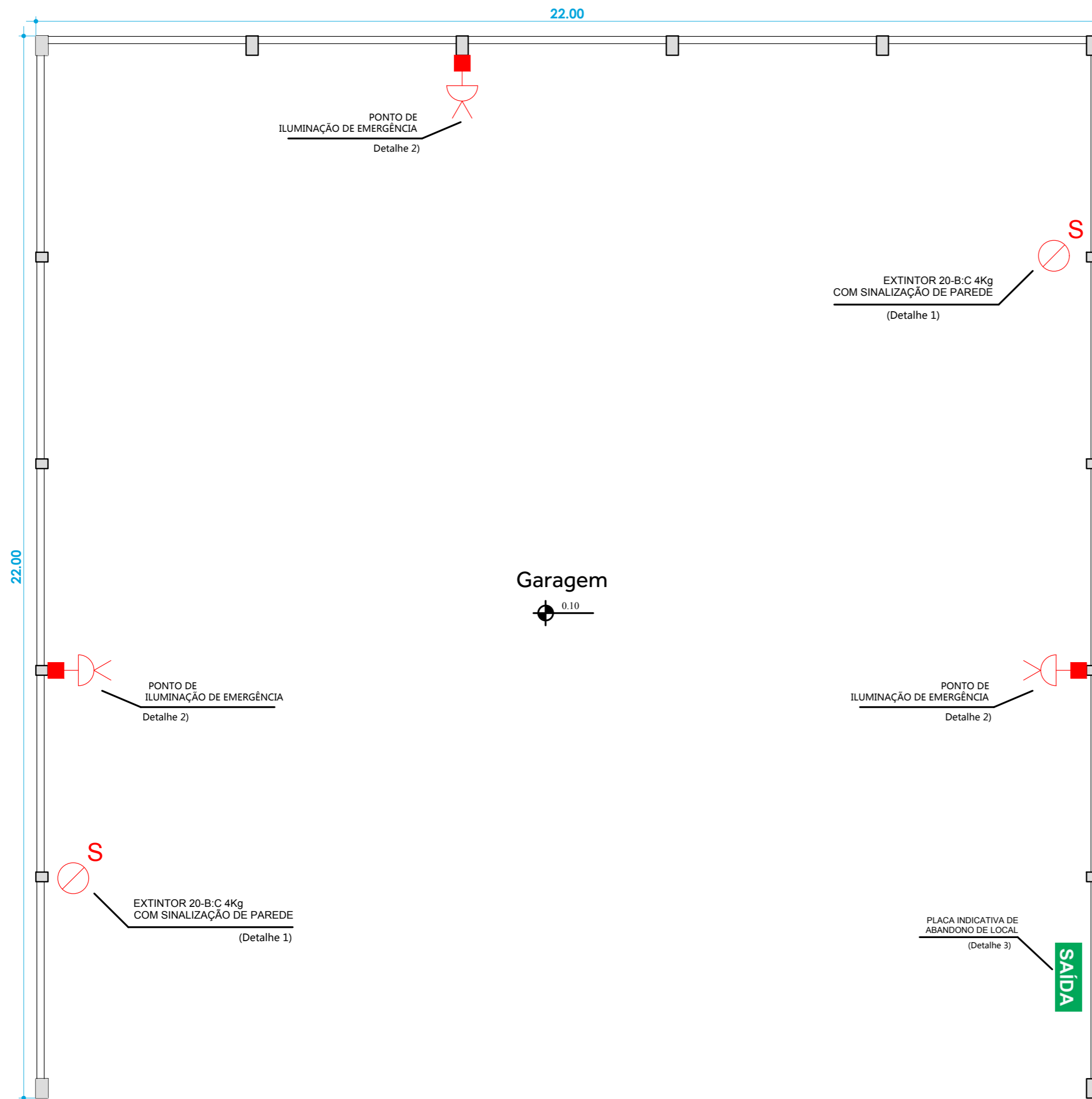
Planta Baixa Galpão | Área: 484,00m 2 | Esc: 1:75
