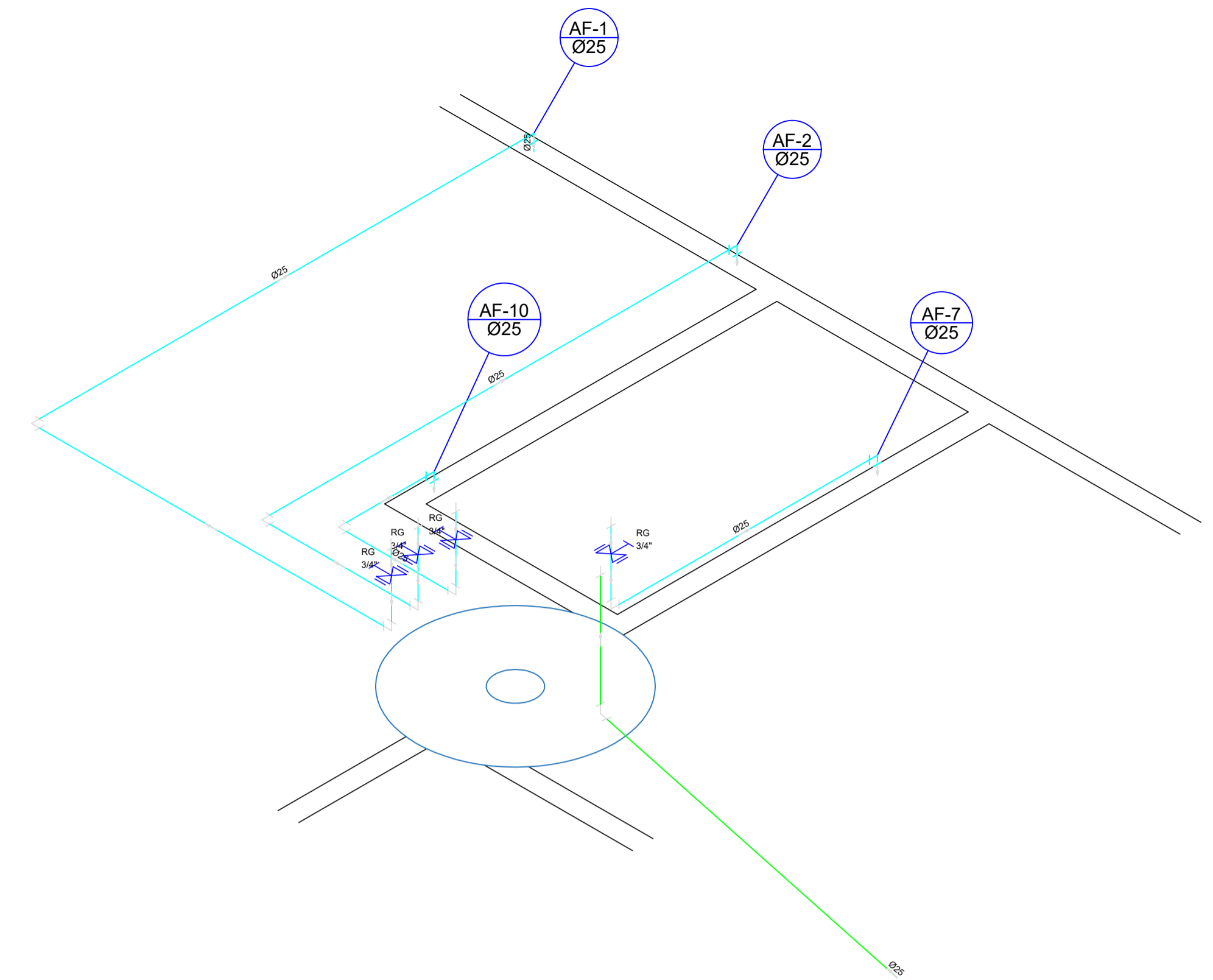
Detalhe H6 escala 1:25
