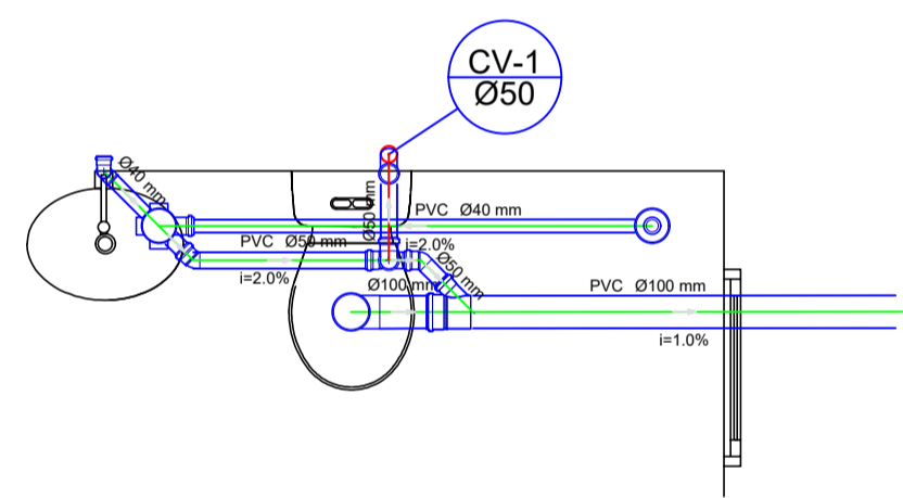
Detalhe S1 escala 1:25
