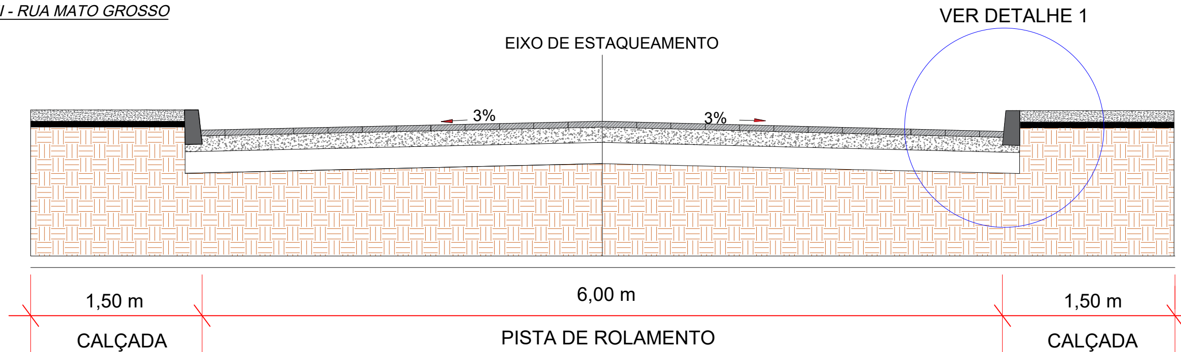
SEÇÃO TIPO II (ESTACAS 8 até 16+3,40) SEM ESCALA
