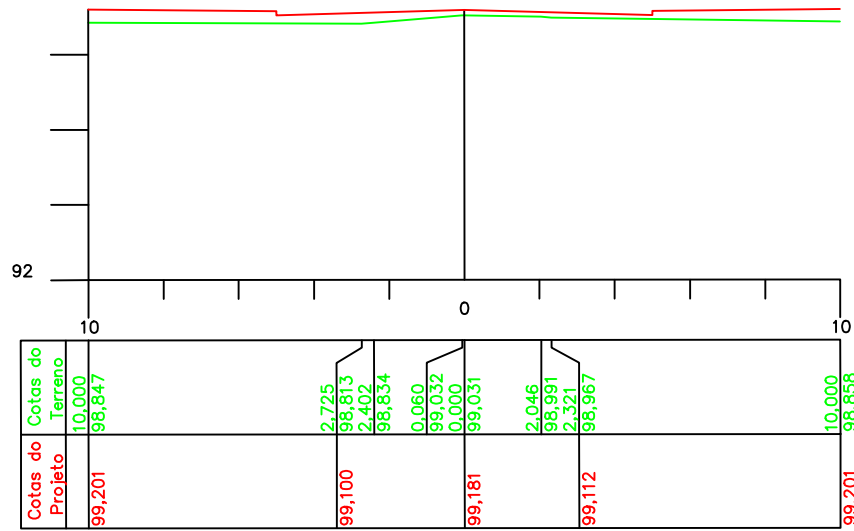
ESTACA 1 Cota do terreno: 99,031 Cota do projeto: 99,181
