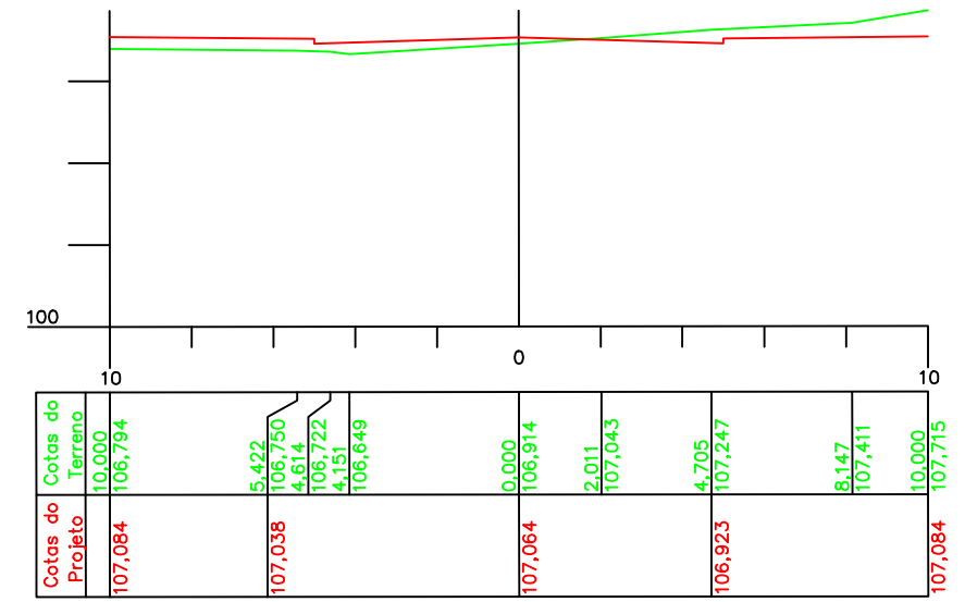
ESTACA 8 Cota do terreno: 106,914 Cota do projeto: 107,064
