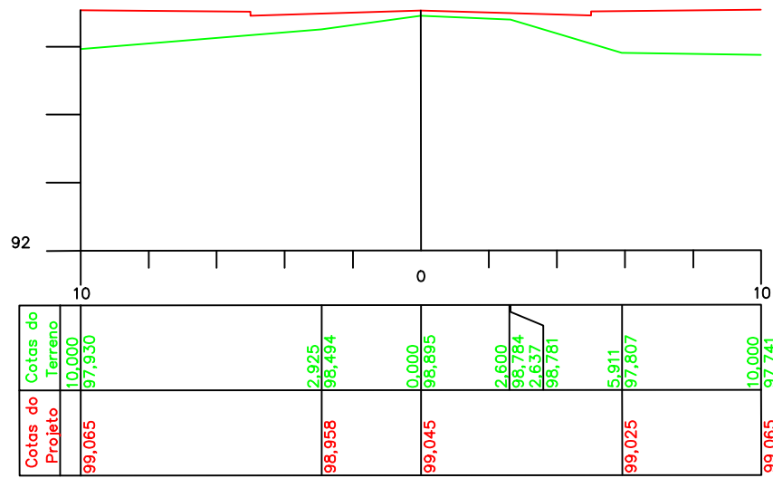
ESTACA 0 Cota do terreno: 99,895 Cota do projeto: 99,045
