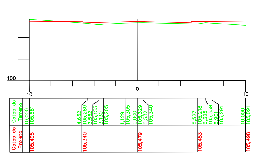
ESTACA 7 Cota do terreno: 105,329 Cota do projeto: 105,479
