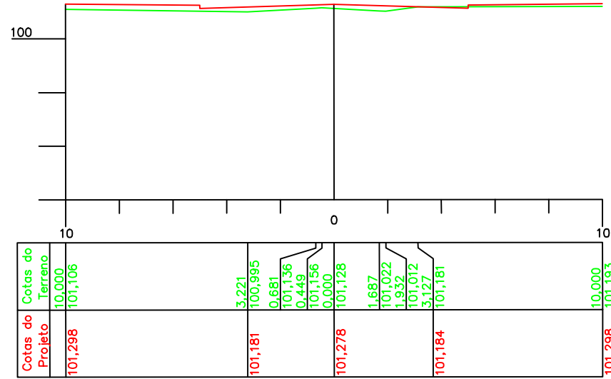
ESTACA 4 Cota do terreno: 101,128 Cota do projeto: 101,278
