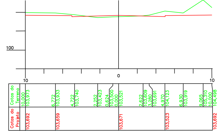
ESTACA 6 Cota do terreno: 103,521 Cota do projeto: 103,671
