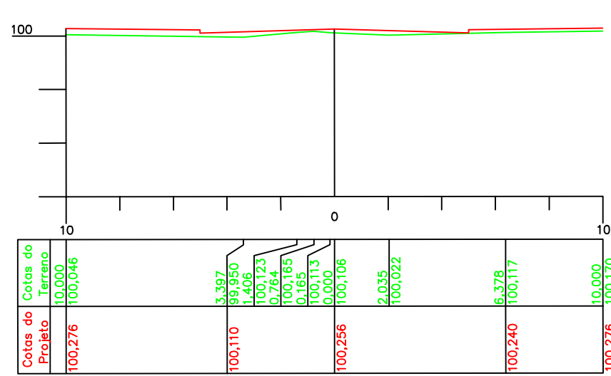
ESTACA 3 Cota do terreno: 100,106 Cota do projeto: 100,256
