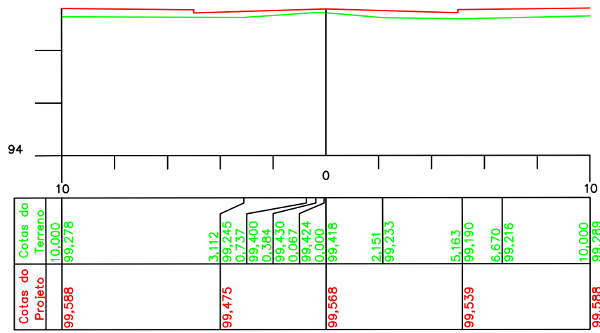
ESTACA 2 Cota do terreno: 99,418 Cota do projeto: 99,568
