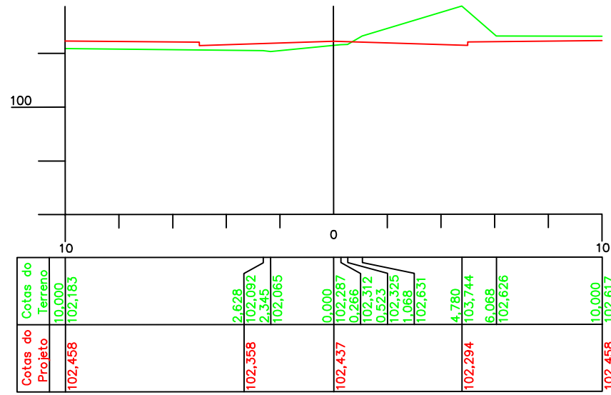
ESTACA 5 Cota do terreno: 102,287 Cota do projeto: 102,437
