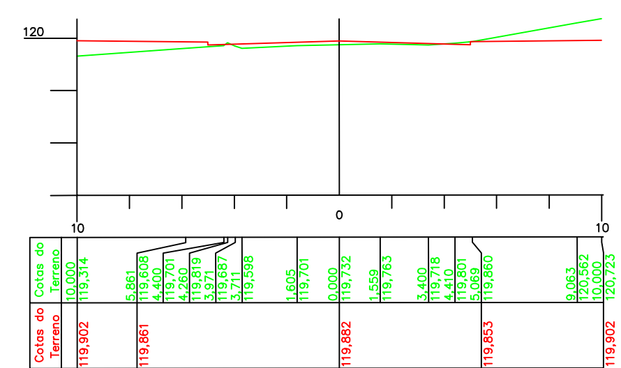
ESTACA 16 Cota do terreno: 119,732 Cota do projeto: 119,882
