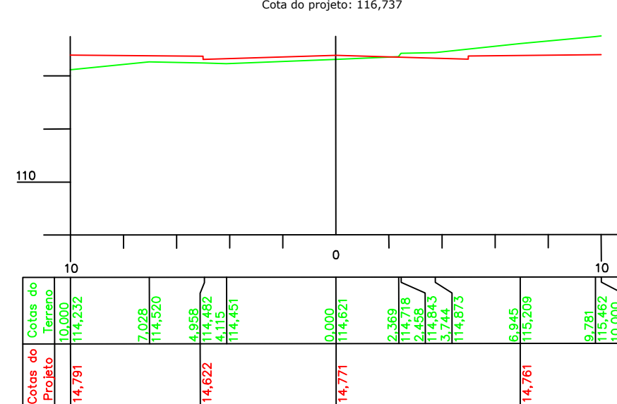
ESTACA 12 Cota do terreno: 114,621 Cota do projeto: 114,771
