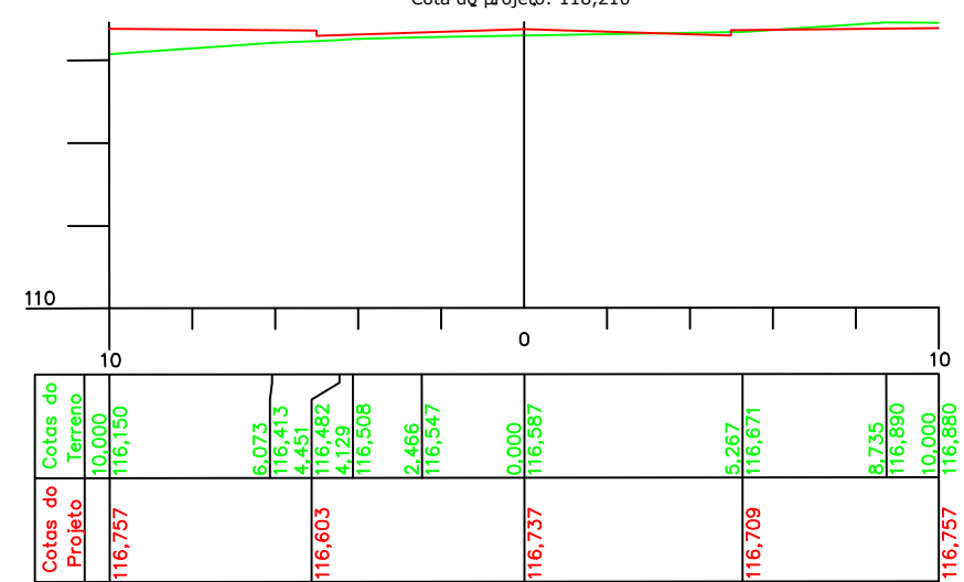
ESTACA 13 Cota do terreno: 116,587 Cota do projeto: 116,737
