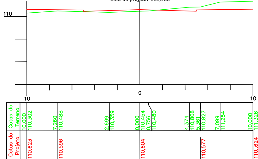
ESTACA 10 Cota do terreno: 110,454 Cota do projeto: 110,604
