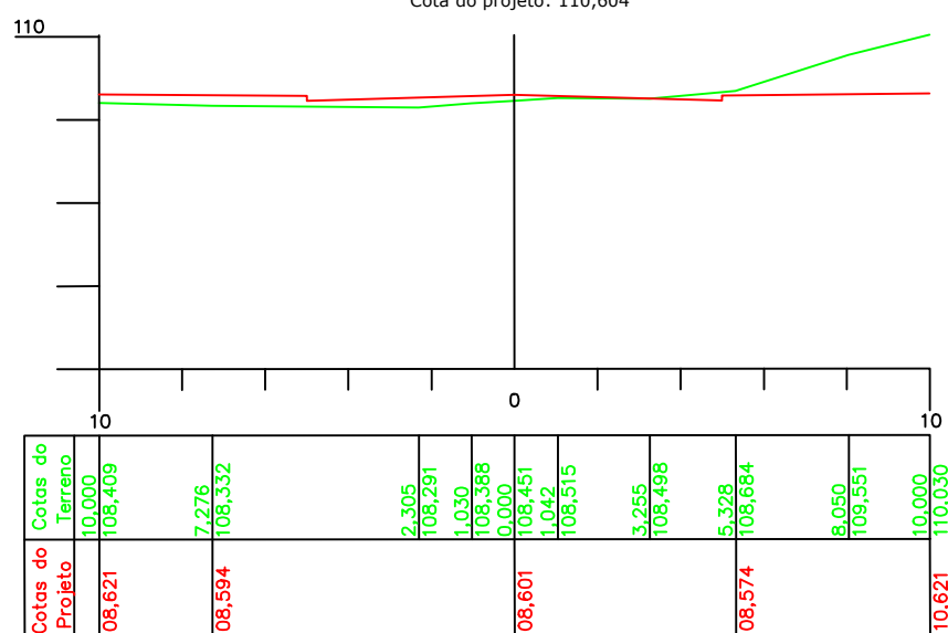
ESTACA 9 Cota do terreno: 108,451 Cota do projeto: 108,601
