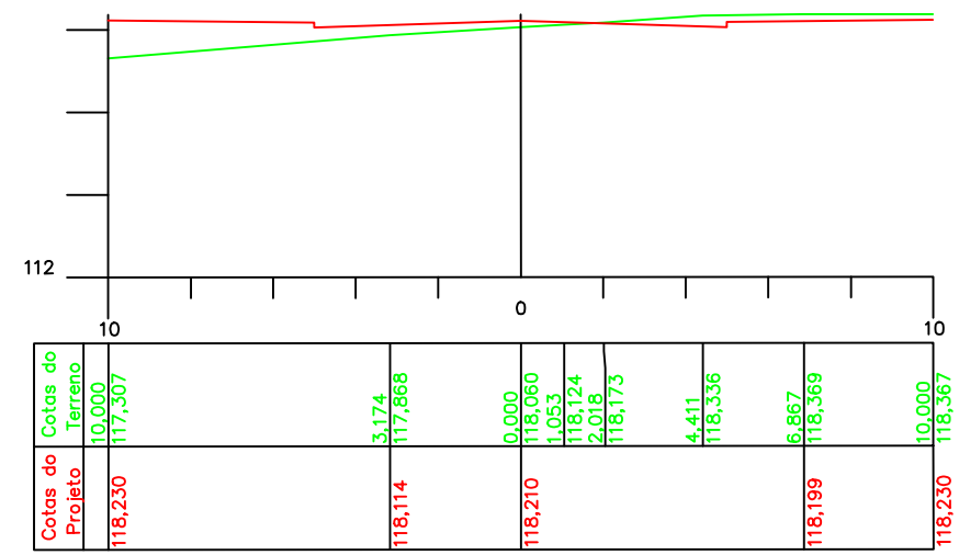
ESTACA 14 Cota do terreno: 118,060 Cota do projeto: 118,210
