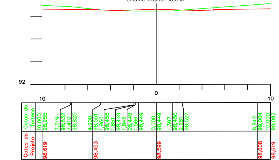
ESTACA 5 Cota do terreno: 98,449 Cota do projeto: 99,599
