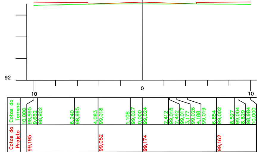
ESTACA 0 Cota do terreno: 99,024 Cota do projeto: 99,174
