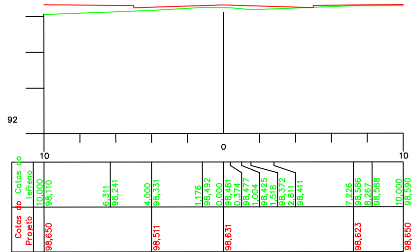
ESTACA 1 Cota do terreno: 98,481 Cota do projeto: 98,631
