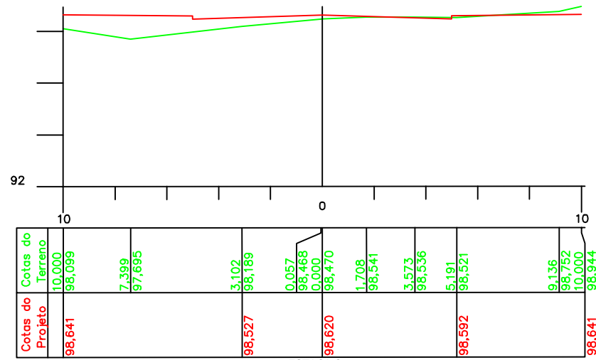
ESTACA 2 Cota do terreno: 98,470 Cota do projeto: 98,620
