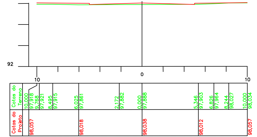
ESTACA 6 Cota do terreno: 97,888 Cota do projeto: 98,038
