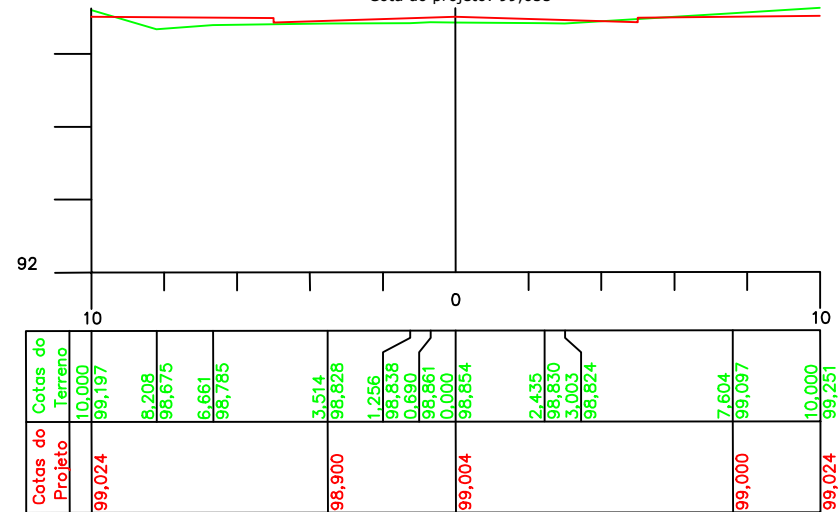
ESTACA 3 Cota do terreno: 98,854 Cota do projeto: 99,004
