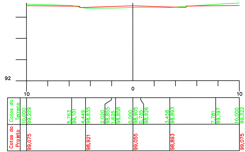
ESTACA 4 Cota do terreno: 98,905 Cota do projeto: 99,055
