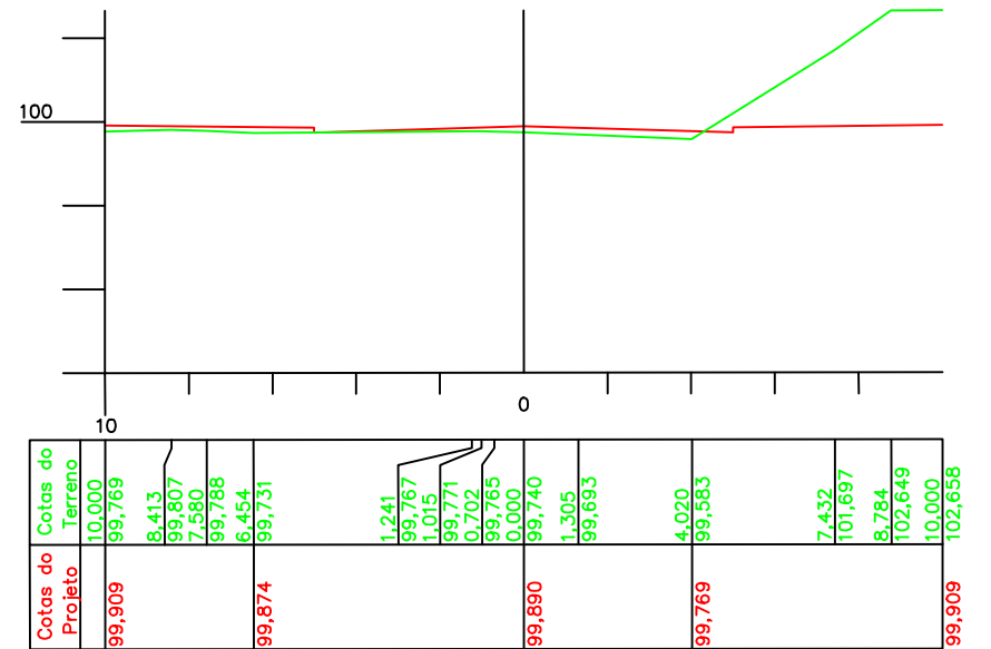
ESTACA 0 Cota do terreno: 99,740 Cota do projeto: 99,890
