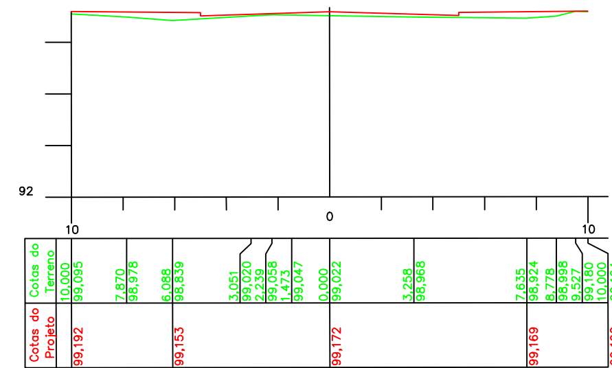
ESTACA 2 Cota do terreno: 99,022 Cota do projeto: 99,172
