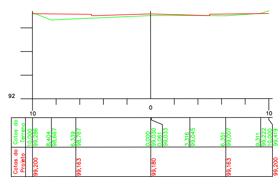
ESTACA 3 Cota do terreno: 99,030 Cota do projeto: 99,180
