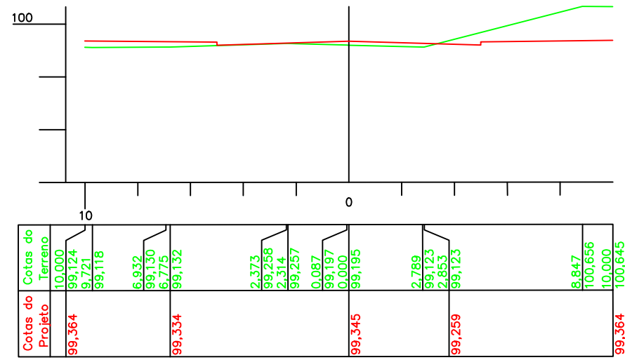
ESTACA 1 Cota do terreno: 99,195 Cota do projeto: 99,345
