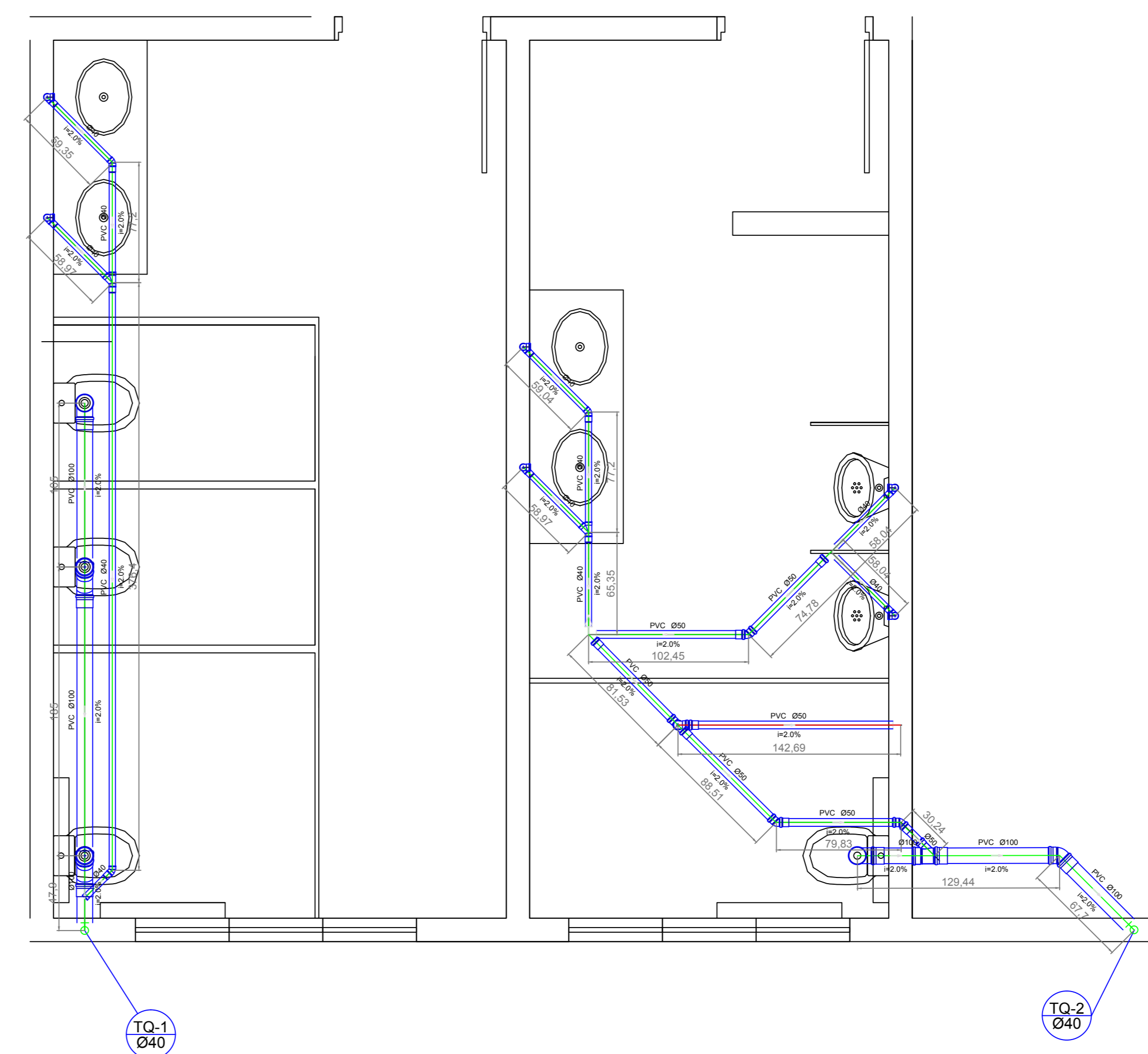
DETALHE S6 ESCALA 1:25
