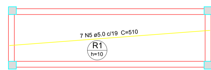
Armação positiva das lajes do pavimento 1.5 (Eixo X) escala 1:50
