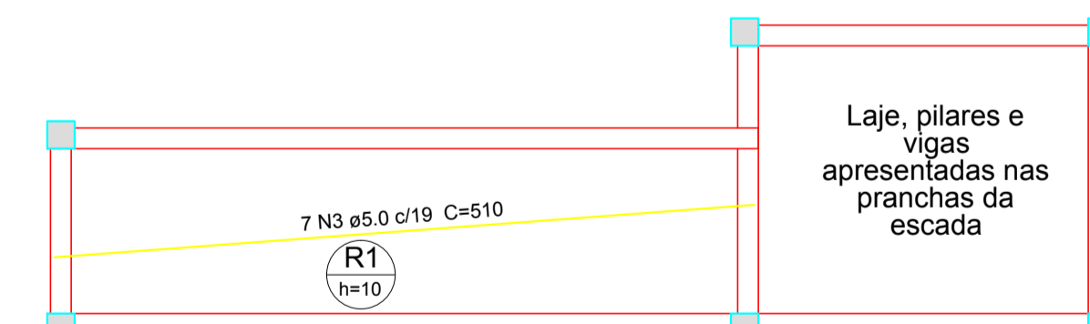
Armação positiva das lajes do pavimento 3 (Eixo X) escala 1:50
