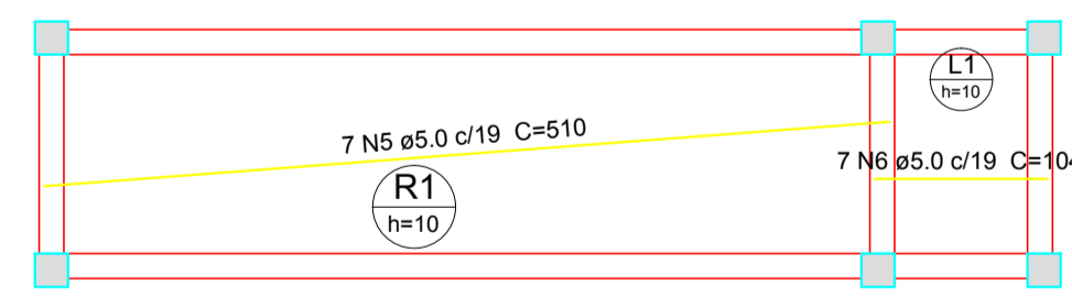
Armação positiva das lajes do pavimento 2 (Eixo X) escala 1:50
