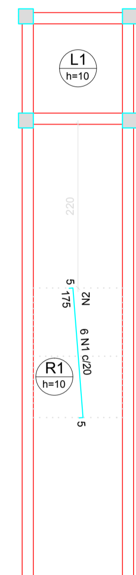
Armação negativa das lajes do pavimento 1 (Eixo Y) escala 1:50
