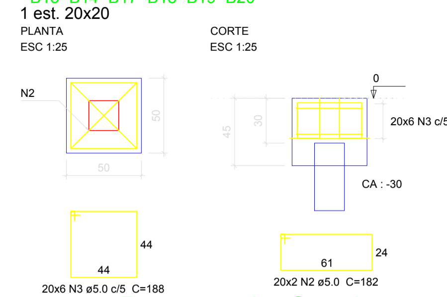
Blocos de fundação escala 1:25
