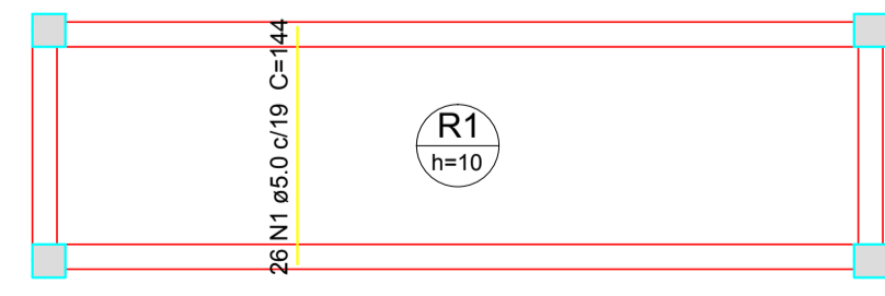
Armação positiva das lajes do pavimento 2.5 (Eixo Y) escala 1:50
