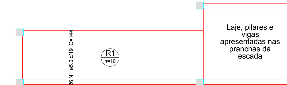
Armação positiva das lajes do pavimento 3 (Eixo Y) escala 1:50
