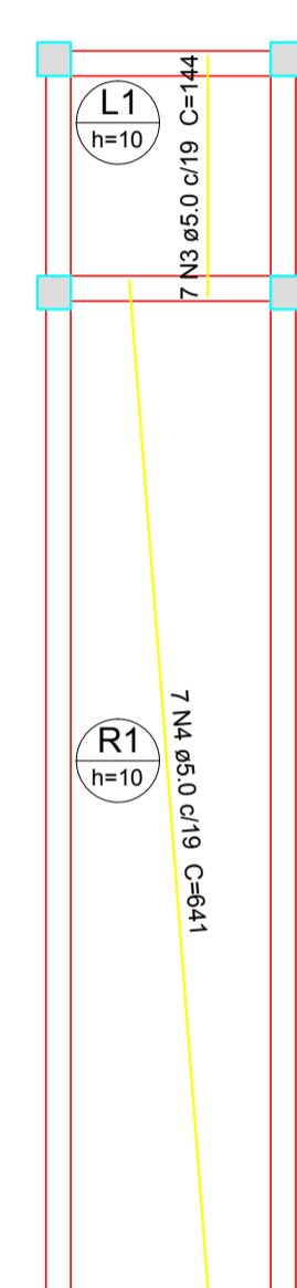
Armação positiva das lajes do pavimento 1 (Eixo Y) escala 1:50
