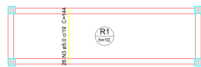
Armação positiva das lajes do pavimento 1.5 (Eixo Y) escala 1:50
