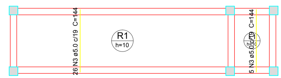
Armação positiva das lajes do pavimento 2 (Eixo Y) escala 1:50
