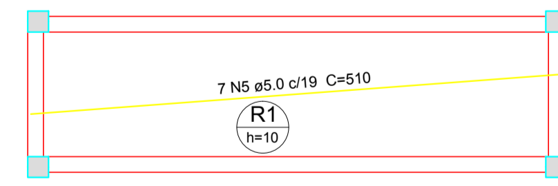
Armação positiva das lajes do pavimento 2.5 (Eixo X) escala 1:50
