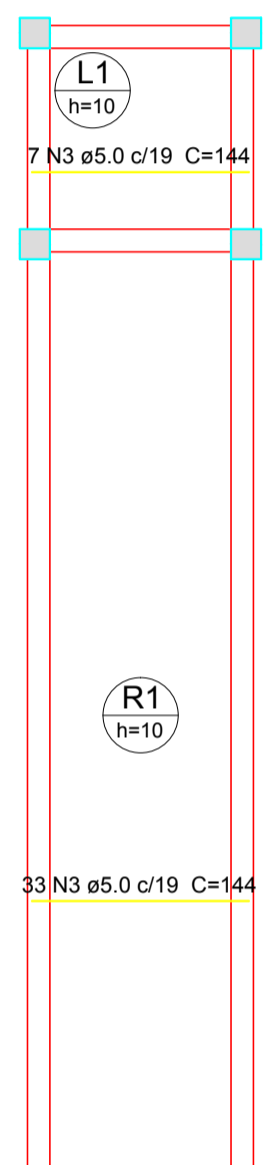
Armação positiva das lajes do pavimento 1 (Eixo X) escala 1:50
