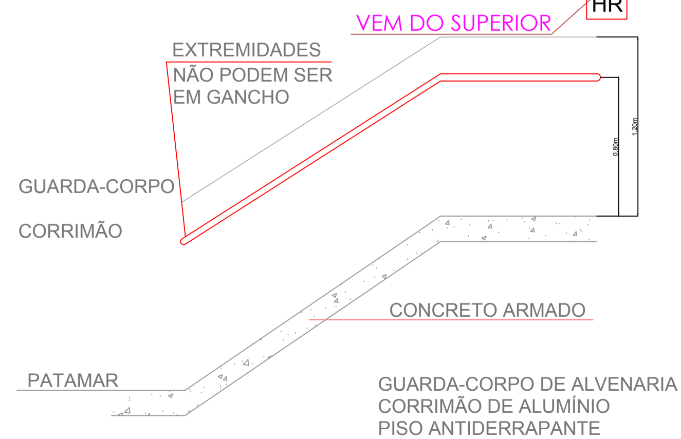
DETALHE CORRIMÃO E GUARDA CORPO sem escala
