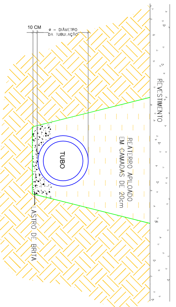
ASSENTAMENTO DE TUBOS
