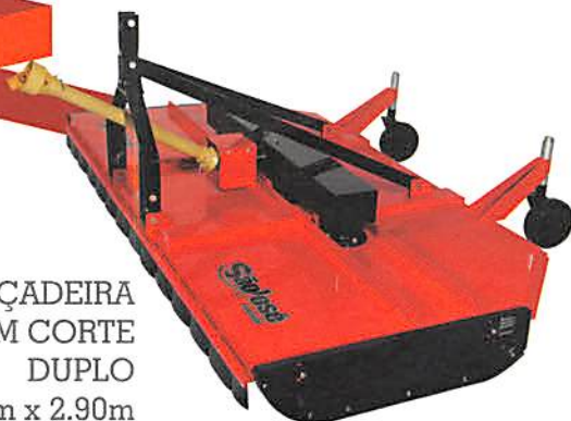
ROÇADEIRA COM CORTE DUPLO 3.5m x 3.5m Ref.262
