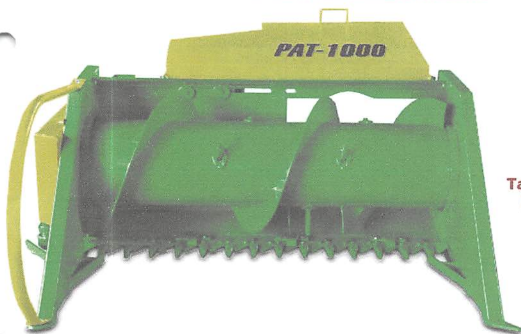
SISTEMA DE TRANSMISSÃO ATRAVÉS DE CORRENTES E CORREIAS
