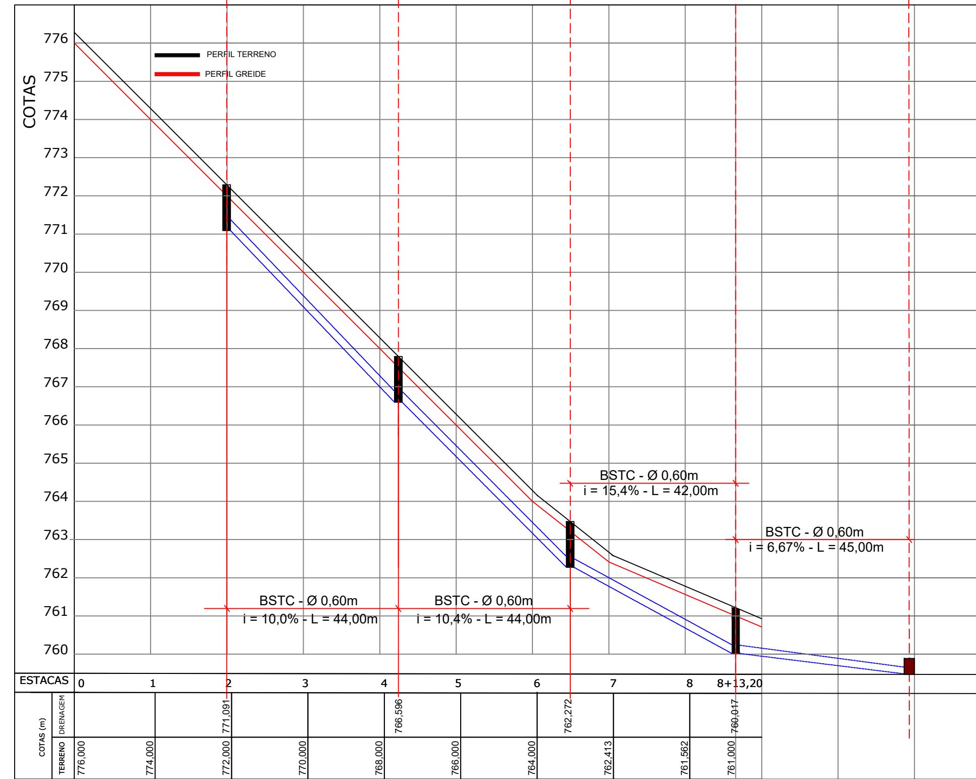
PERFIL LONGITUDINAL Esc. 1/1000
