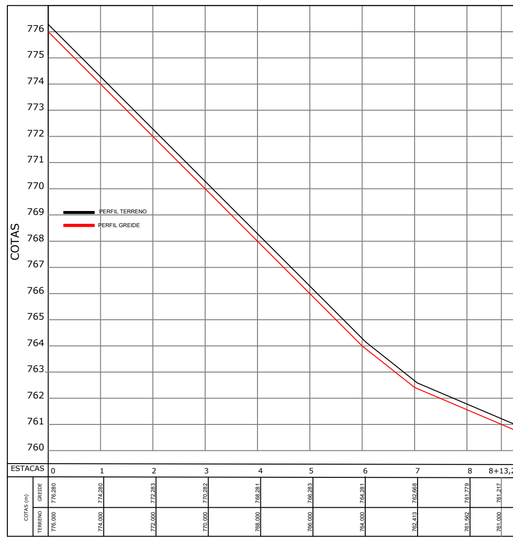
PERFIL LONGITUDINAL Esc. 1/1000
