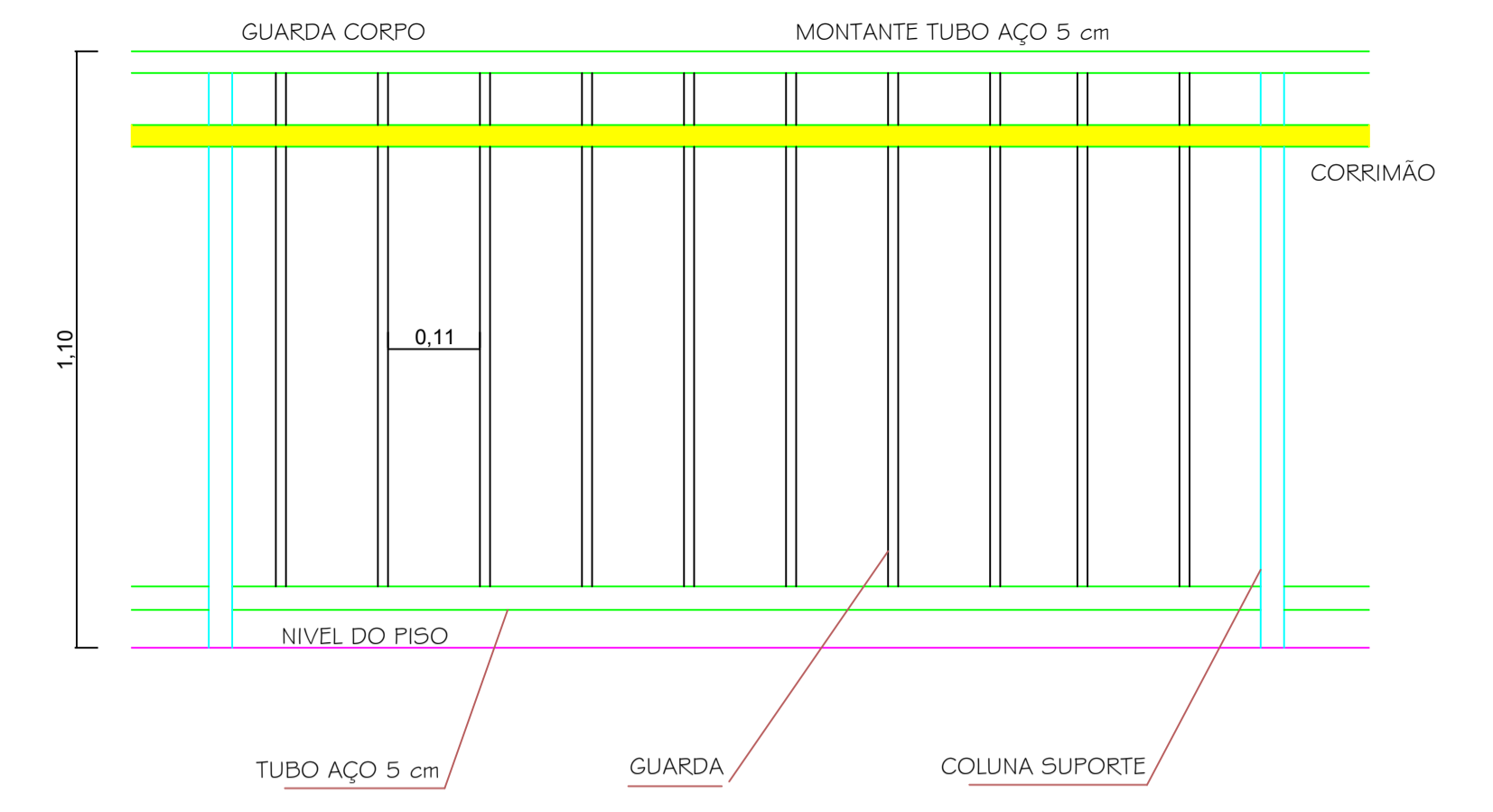
Detalhe Guarda Corpo S/ Escala
