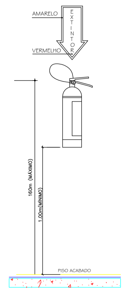
DETALHES DO EXTINTOR DE INCÊNDIO COM SINALIZAÇÃO DE PAREDE S/ Esc.
