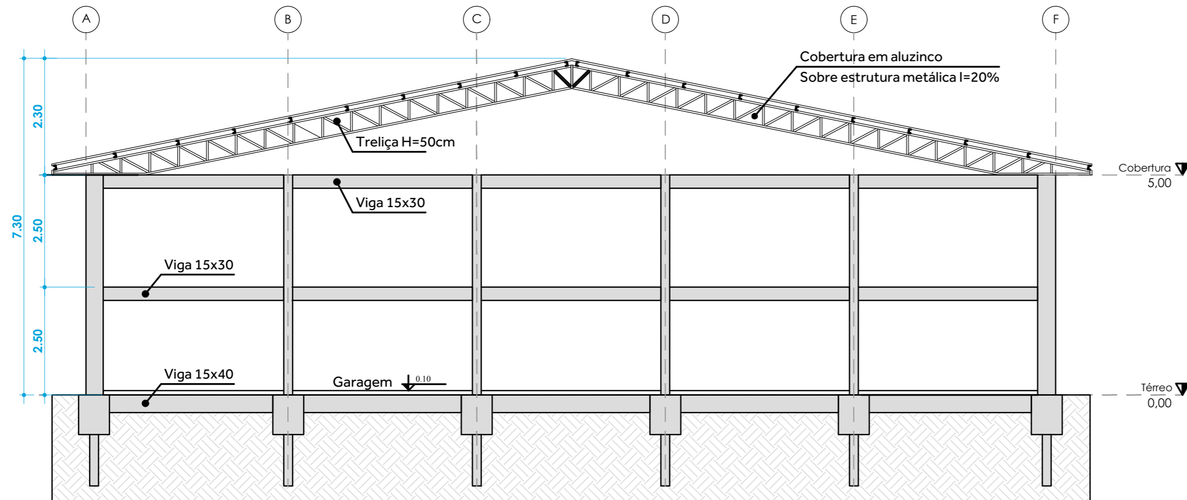
Corte A | ESC: 1:75
