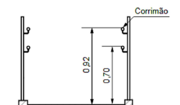
Detalhe 04 - Corrimão
