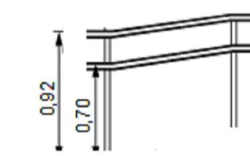
Detalhe 03 Corrimão com suporte vertical
