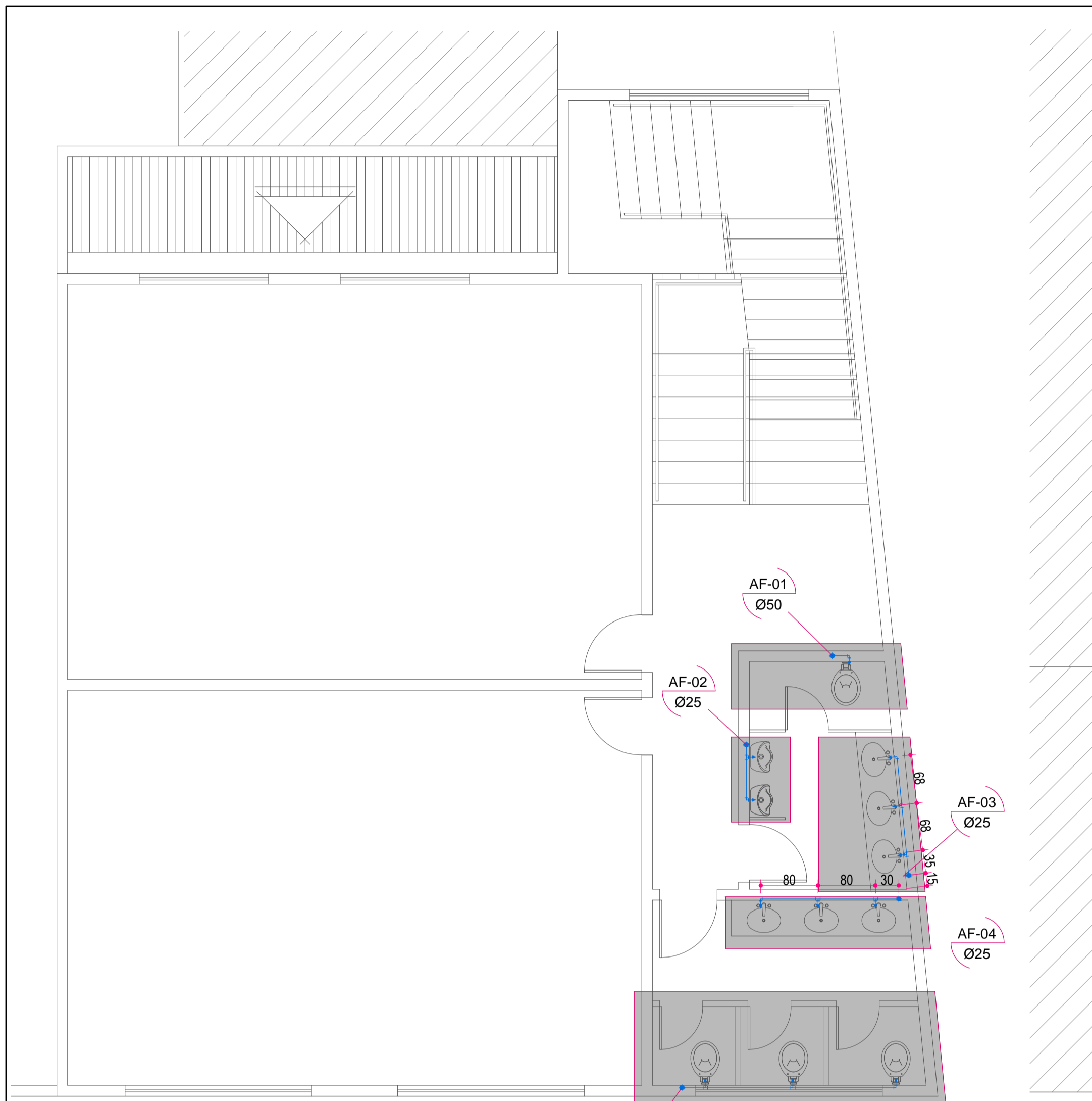
1.0 PLANTA BAIXA 1 PV. ESCALA 1:50
