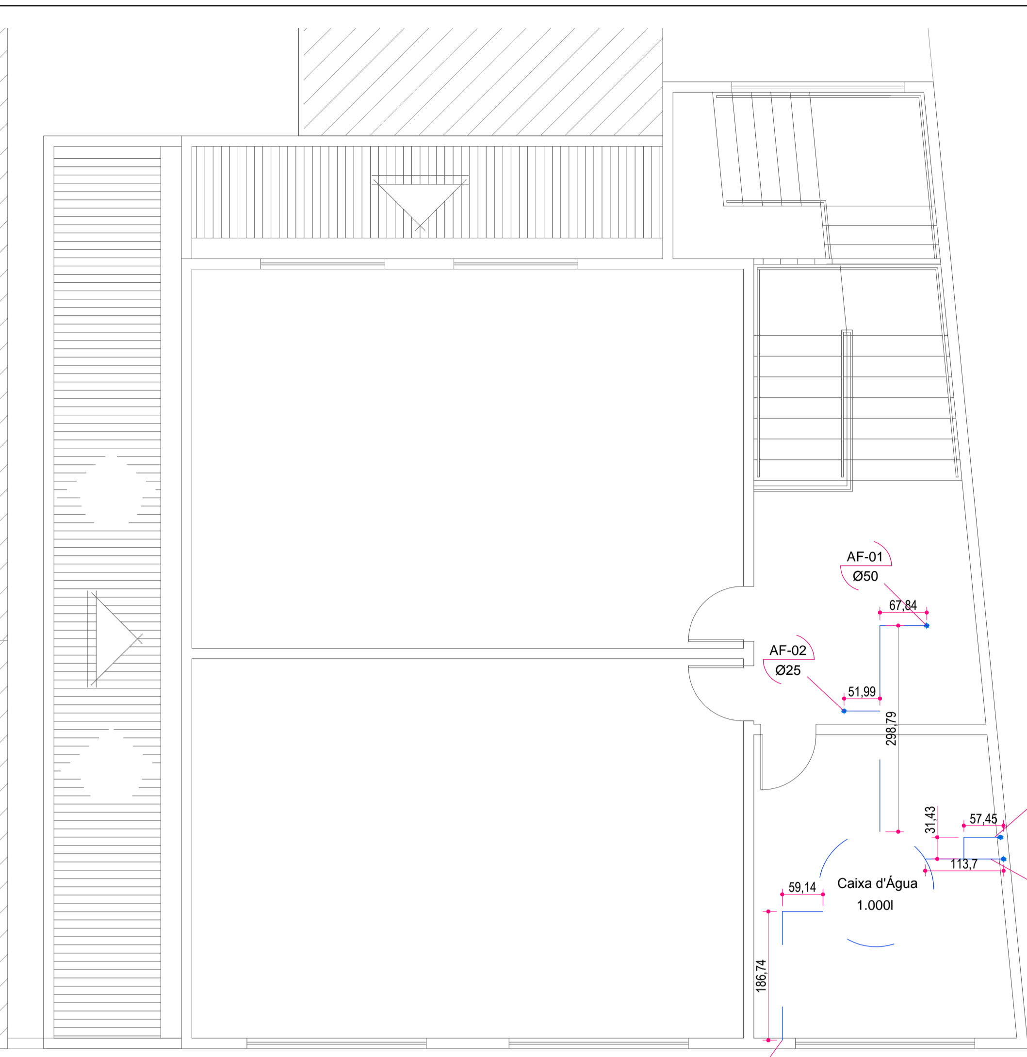
1.1 PLANTA BAIXA 2 PV. ESCALA 1:50
