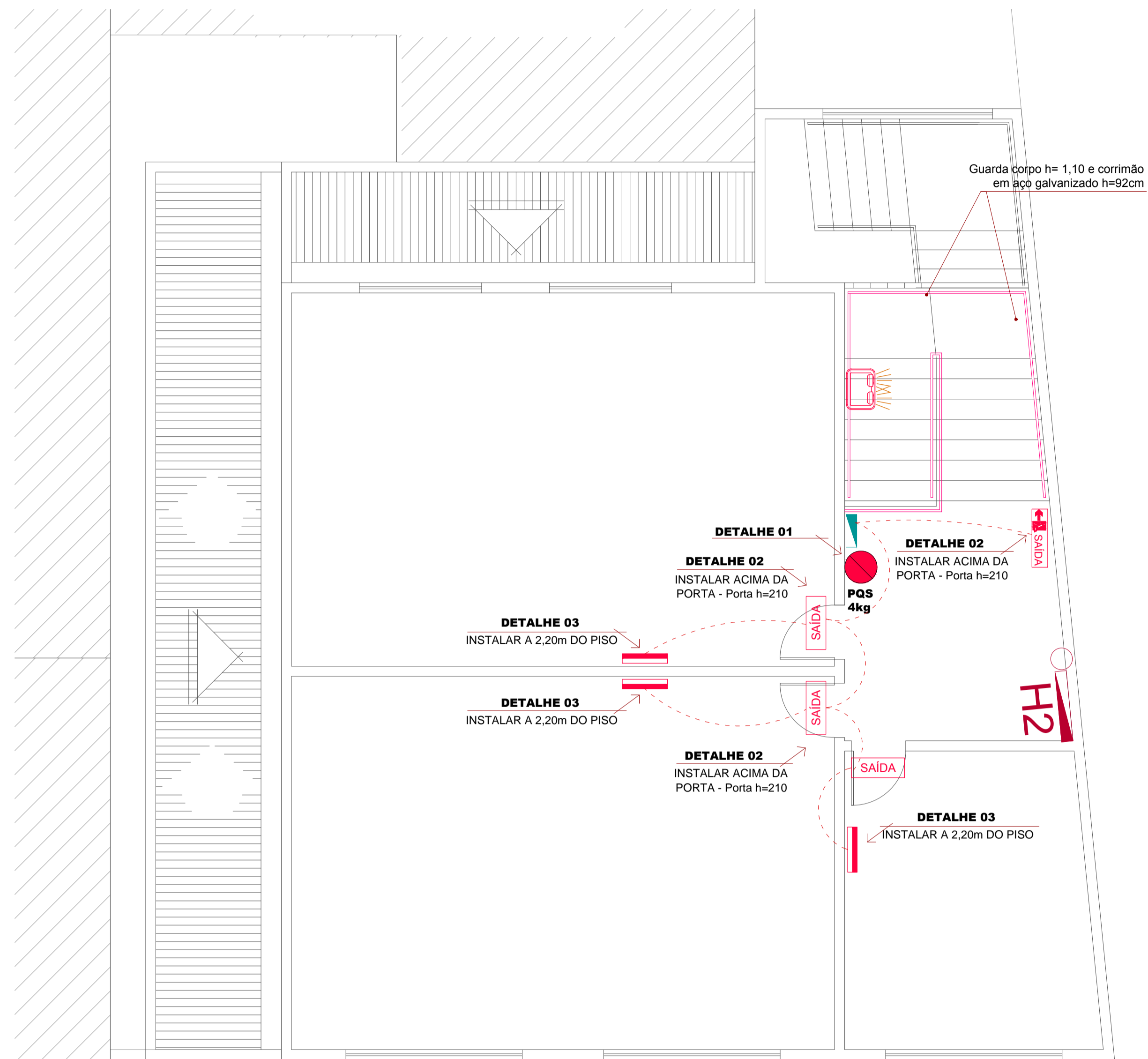
1.2 PLANTA BAIXA 2 PV. ESCALA 1:50
