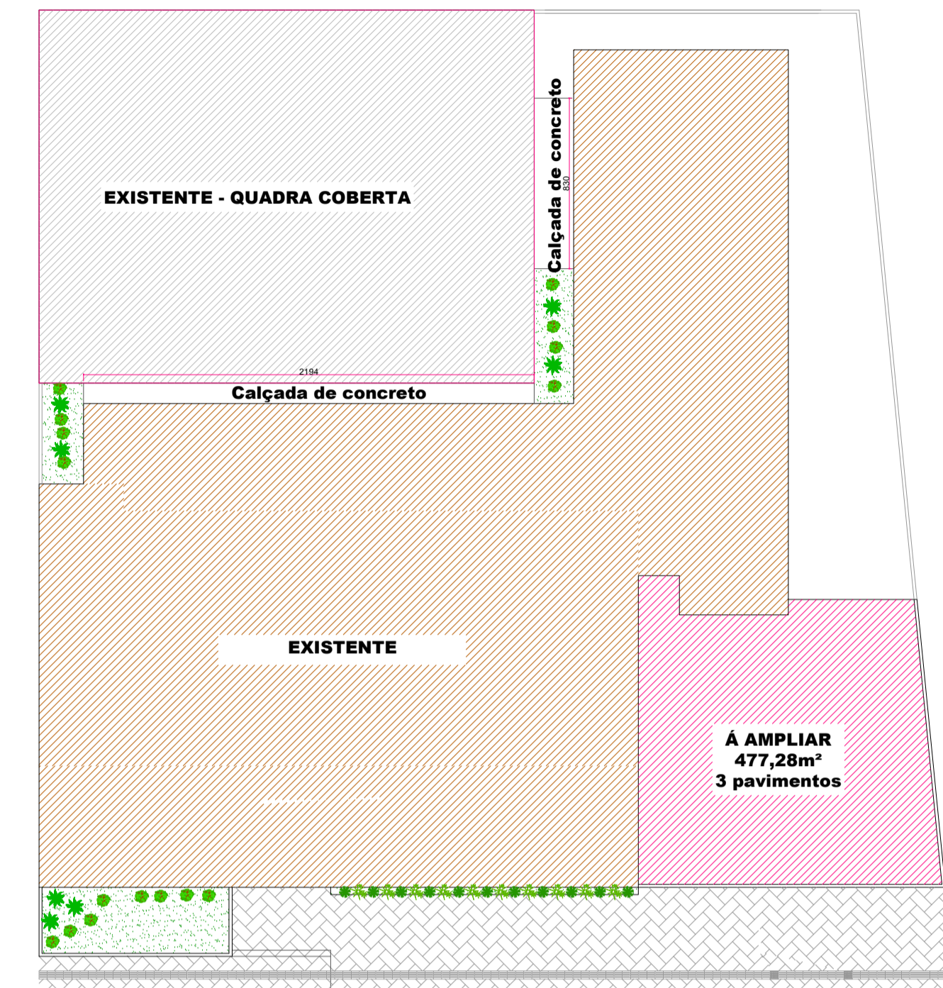
1.0 IMPLANTAÇÃO ESCALA 1:250
