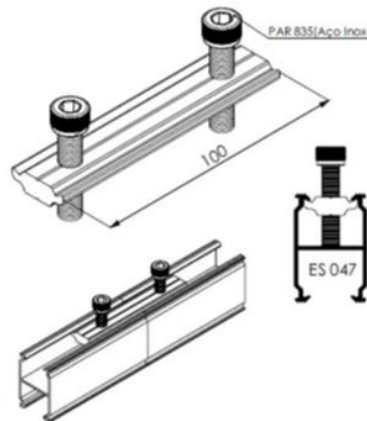
SUP 944 CONEXÃO PARA O PERFIL ES 047 / ES 062 / ES 066 / ES 068
