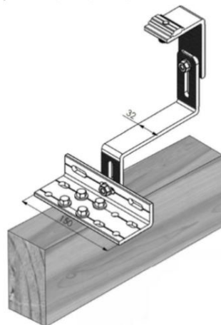
SUP 940 SUPPORTE GANCHO PARA TELHA CERÂMICA Para perfis ES 047 / ES 066 / ES 099 / ES 100
